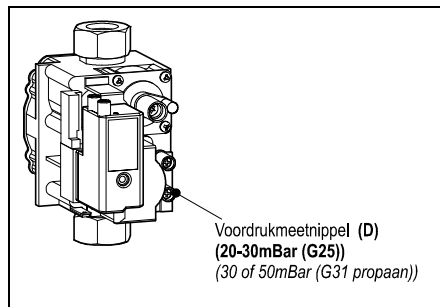
Voordrukmeetnippel (D) (20-30mBar (G25)) (30 of 50mBar (G31 propaan))
